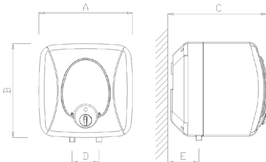
fig.-1 – Model APARICI SB15
