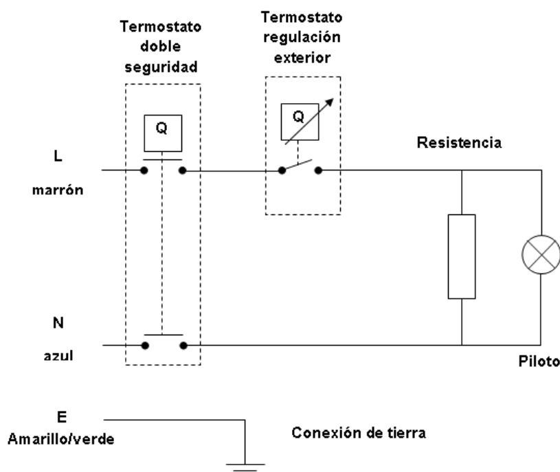
Fig. – 4 Schema modello APARICI – SB15
