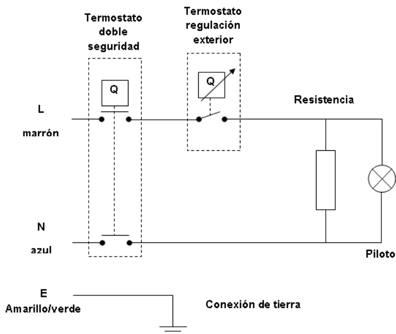
Fig. – 4 Esquema unifilar modelo APARICI – SB15
