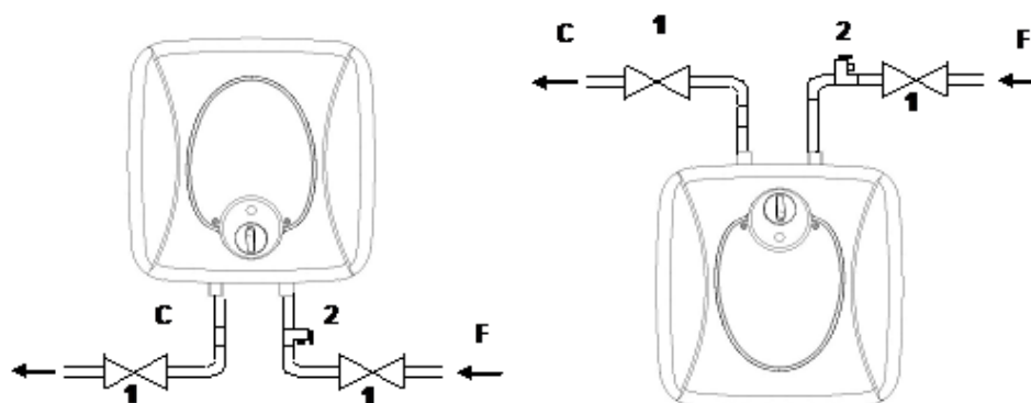
Fig-3 Installazione idraulica
