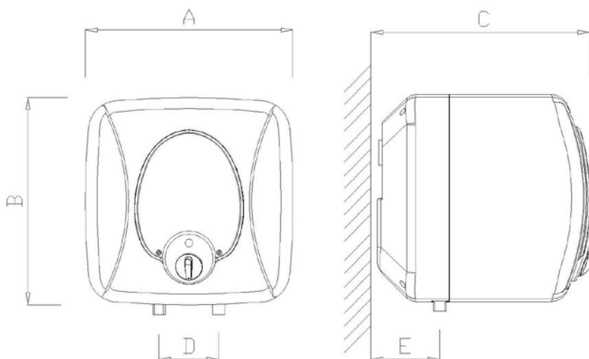
fig.-1 – Modelo APARICI SB15
