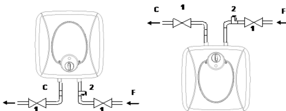
Fig-3 Installazione idraulica
