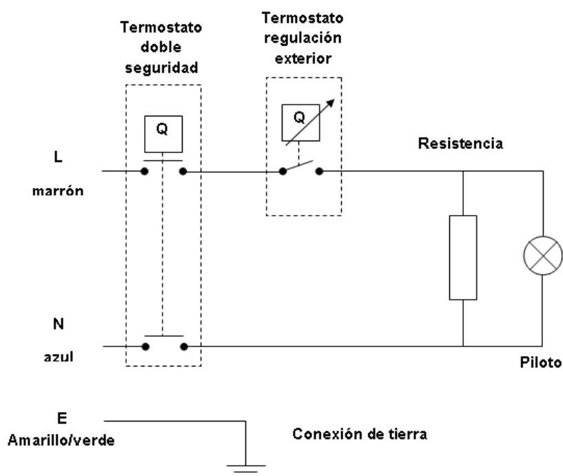
Fig. – 4 Esquema unifilar modelo APARICI – SBxxxN
