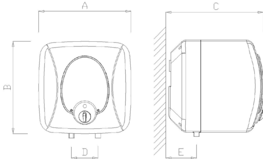
fig.-1 – Modelo APARICI SB15
